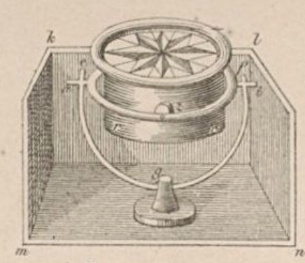
Steuer-Kompass.
