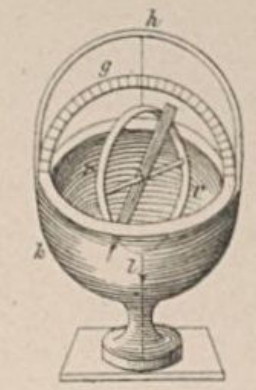
Inklinatorium.
